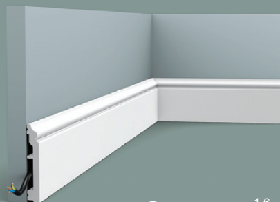
SX173 200 x 10 x 1,6 cm Duropolymer®
