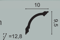
CB512N 200 x 9,5 x 10 cm Durofoam®
